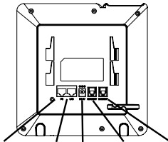
PC-Anschluss LAN-Anschluss Netzanschluss Kopfhörer-Anschluss Hörer-Anschluss
